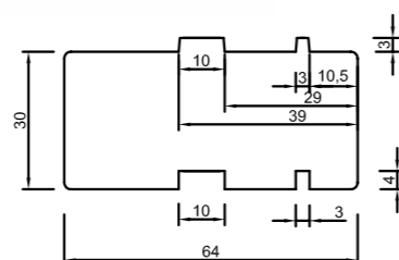
WKŁADKA TERMICZNA POD PRÓG ALUMINIOWY
