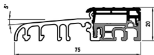
PRÓG ALUMINIOWY Z WKŁADKĄ TERMICZNĄ
